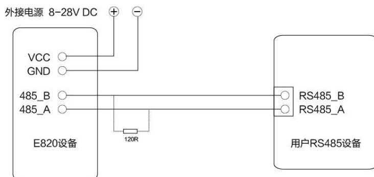
RS485接线图
